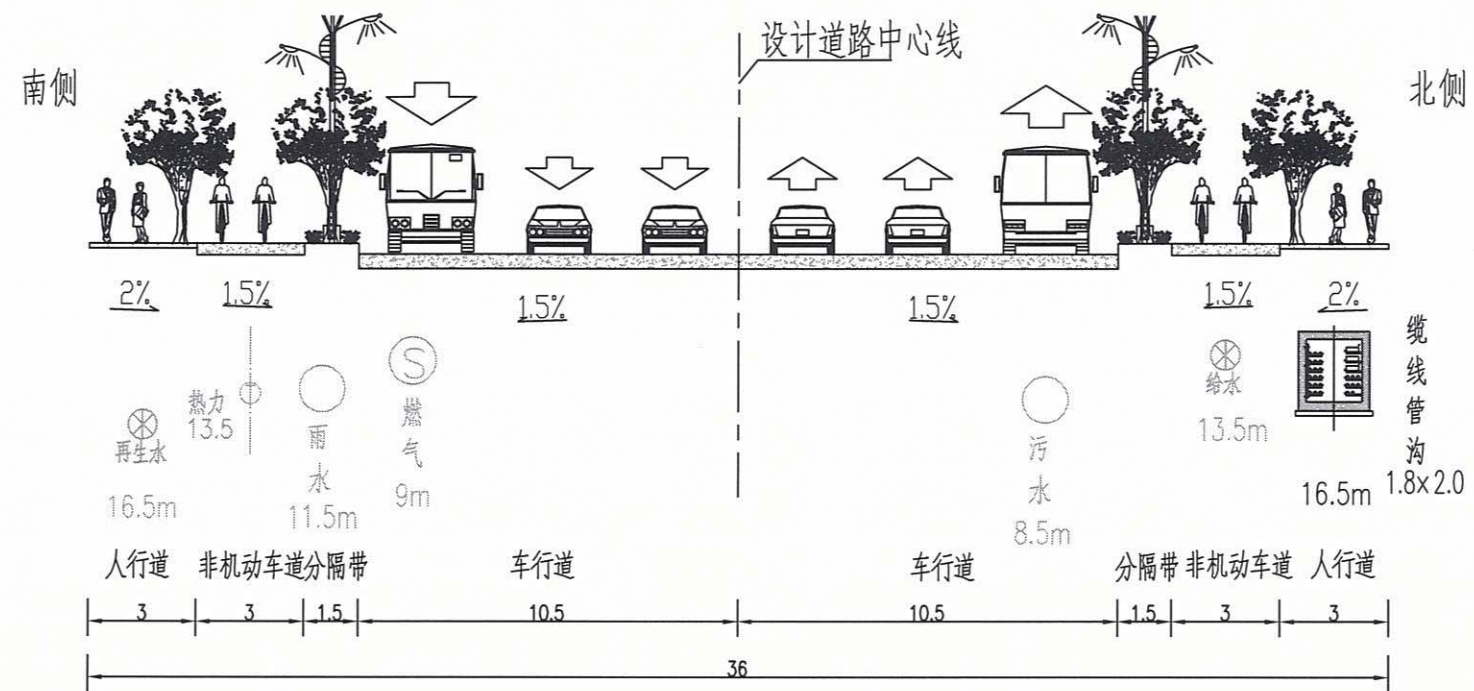
原批复管位横断面示意图
