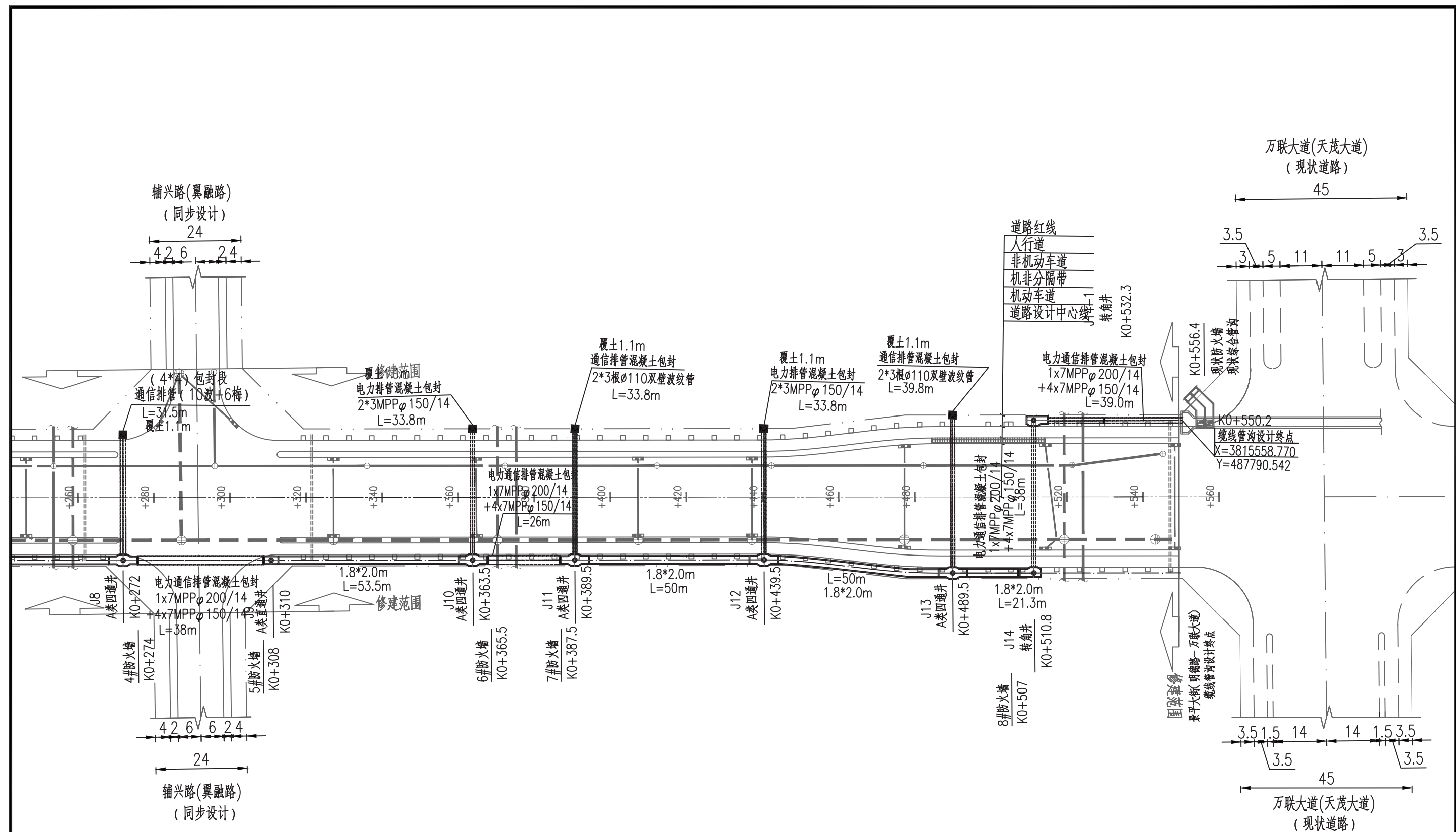
缆线管沟平面图(一)
