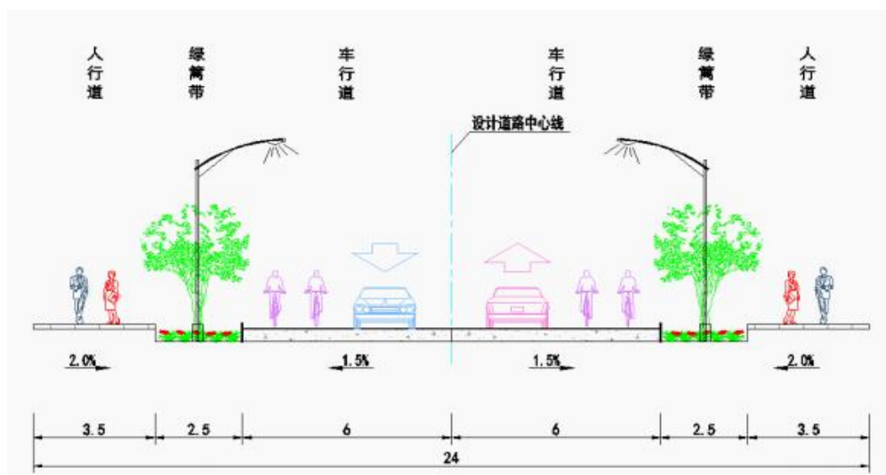
图 2 翼融路道路横断面设计图
