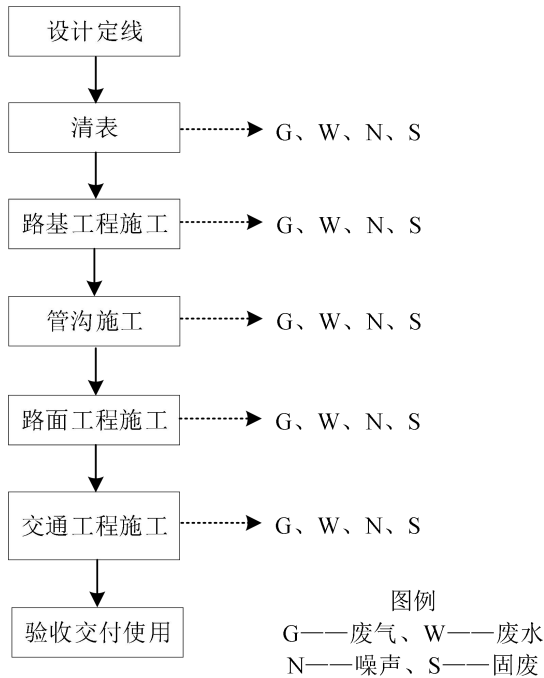
图 5 施工期工艺流程及产污环节
