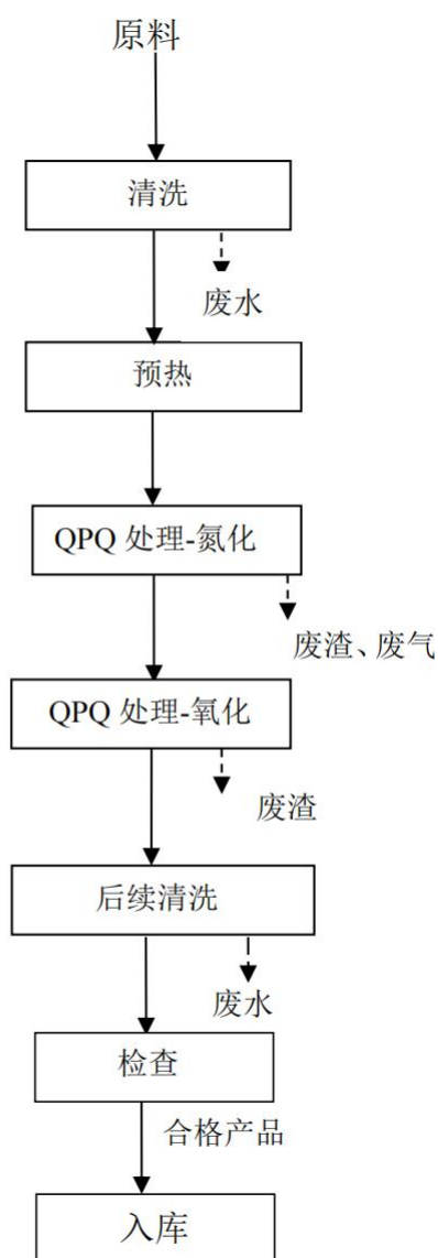
图 2-2 工艺流程图
