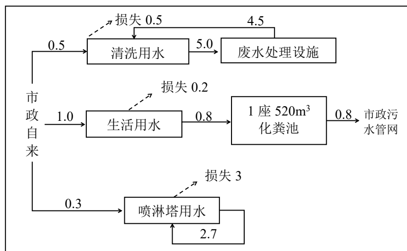
图 2-1 本项目水平衡图 \text{m}^3/\text{d}
