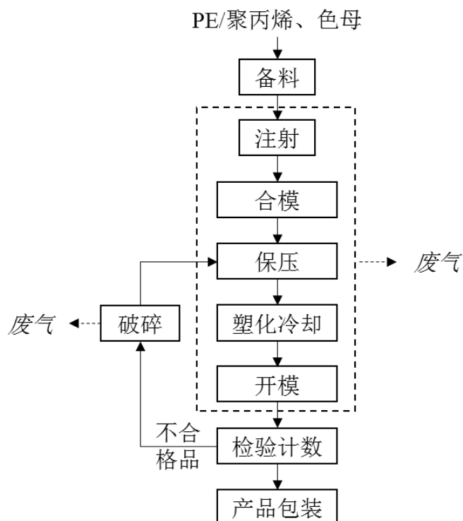
图2-4 项目塑料瓶盖生产工艺流程及产污环节
