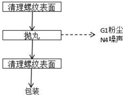
图 2-3 表面处理生产工艺及产污流程图
