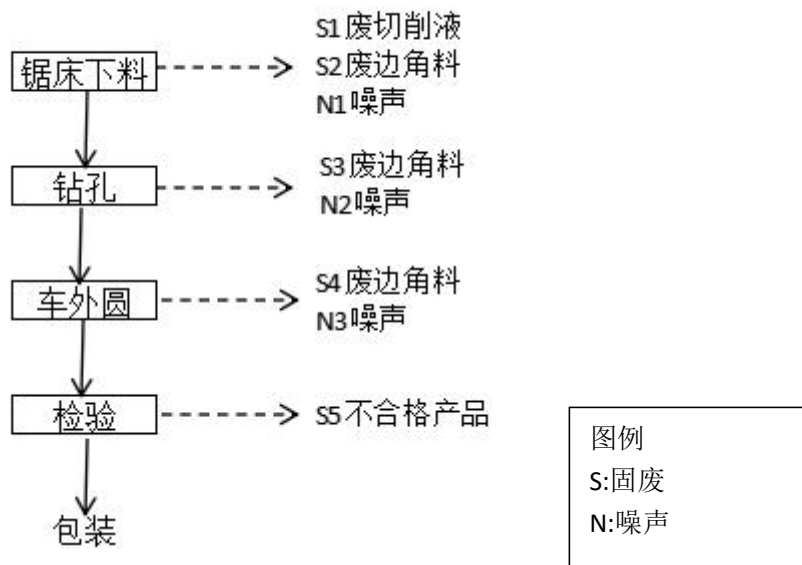
图 2-2 机加工生产工艺及产污流程图
