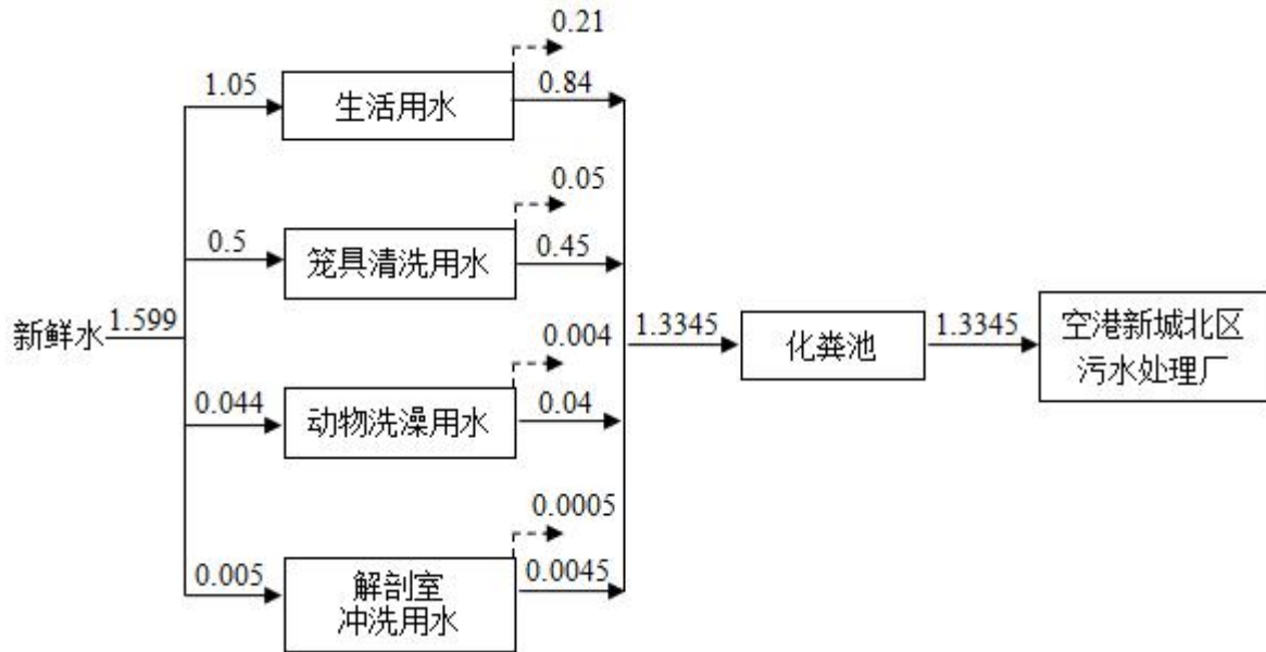
图 2 项目水平衡图 单位：m³/d
